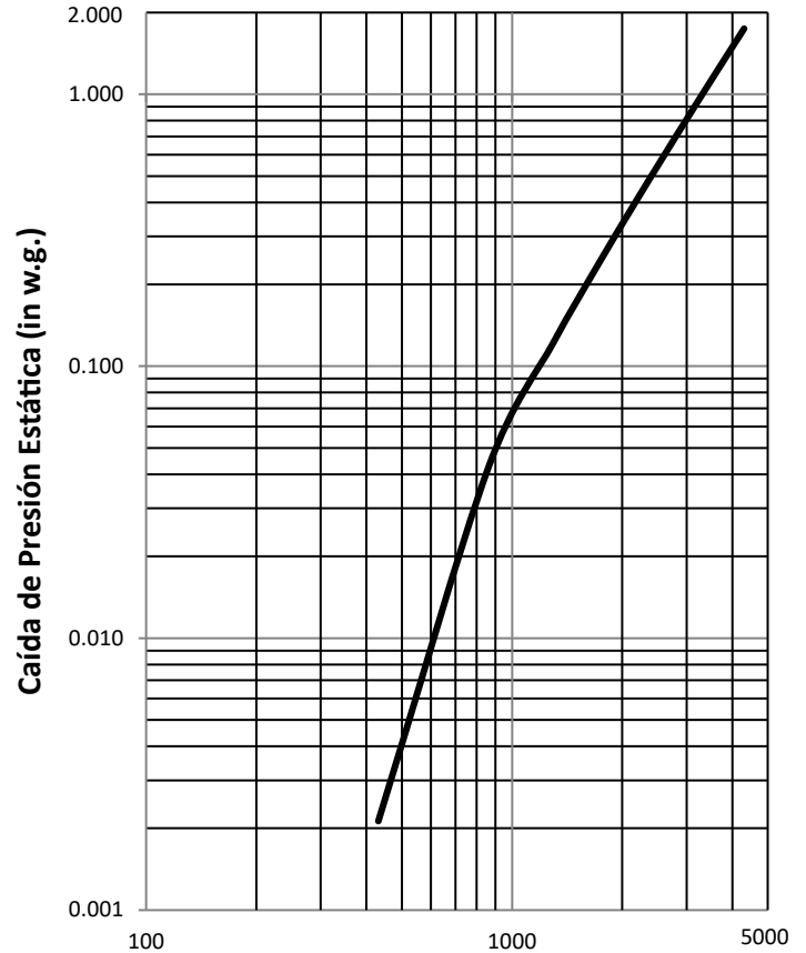
COMPUERTA CBAD (TAMAÑO 12"x12")
