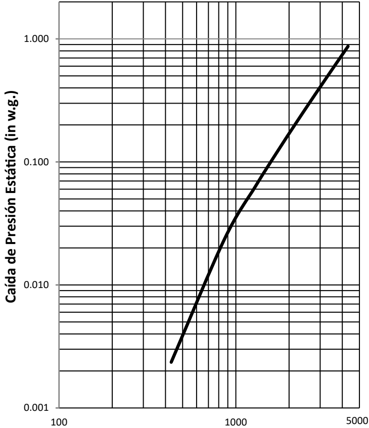
COMPUERTA CBAD (TAMAÑO 36"x36")
