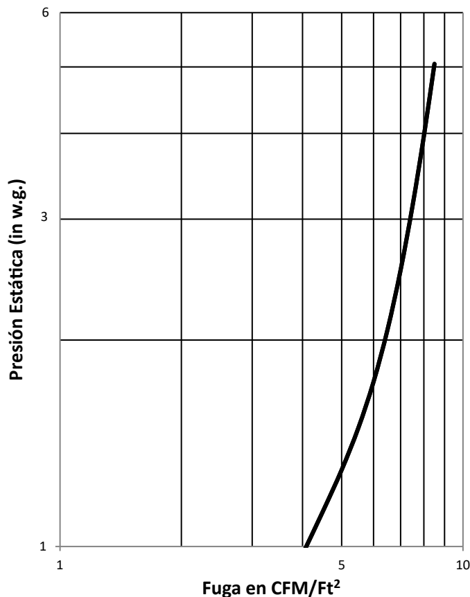
COMPUERTA CBAD (TAMAÑO 12"x12")
