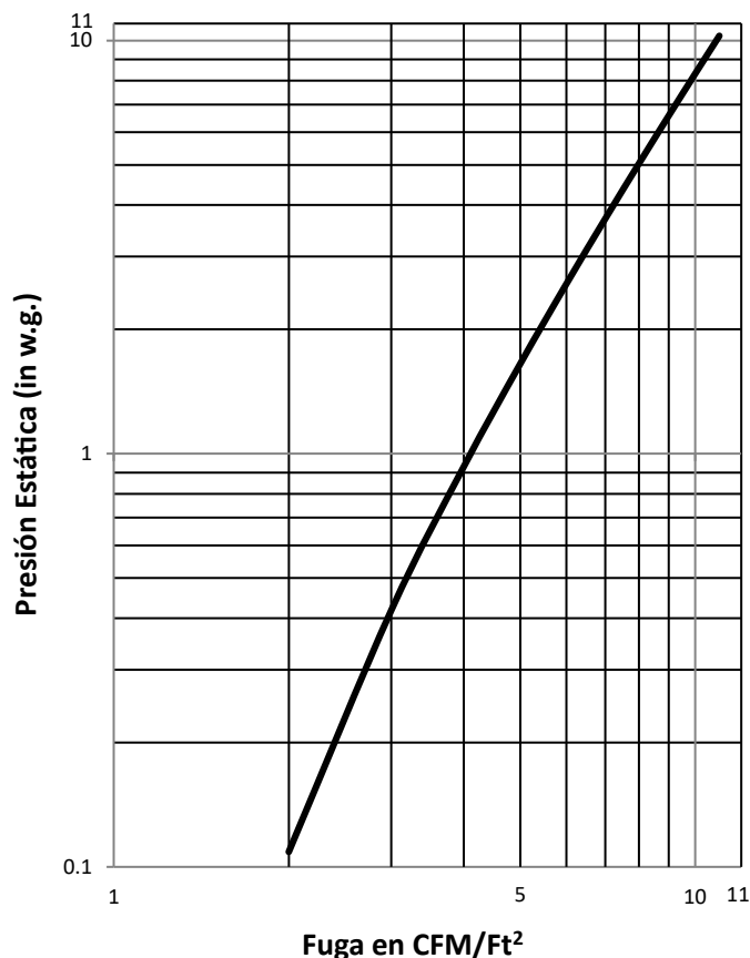
COMPUERTA CBAD (TAMAÑO 48"x36")
